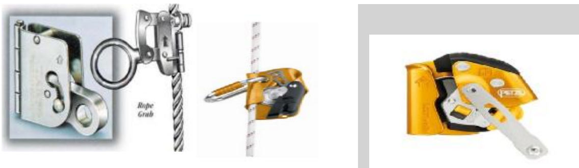
شکل 20 - گیره متوقف کننده سقوط (گیره طناب)
