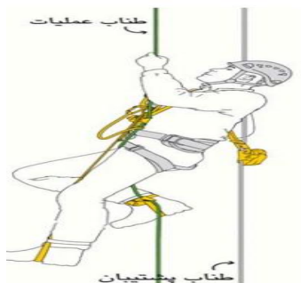
شکل 16- نحوه استفاده از طناب عملیات و طناب پشتیبان
